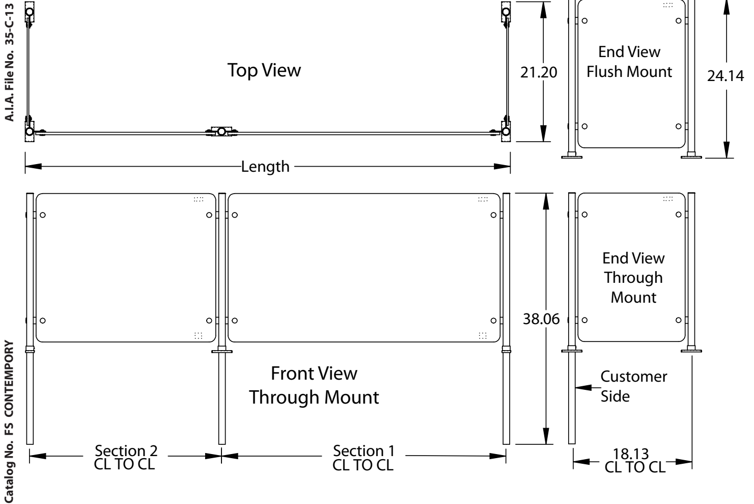
TS412-74 Shown Above
